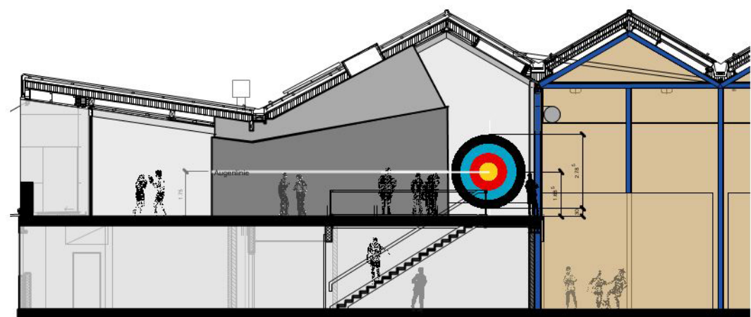
Schnitt A-A 1:50
