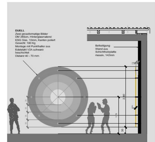
Schnitt B-B 1:50
